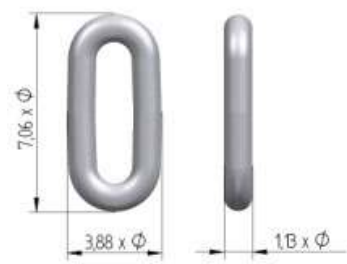
End Link
